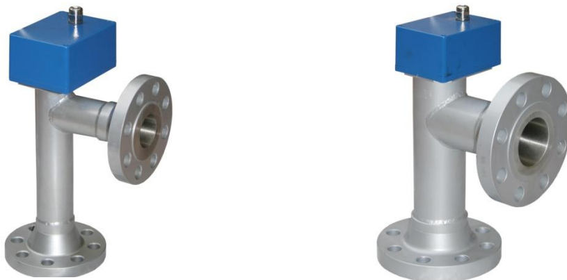
Первичный измерительный преобразователь влагомеров ВСН-2-50-01 и ВСН-2-80-01 в угловом исполнении
